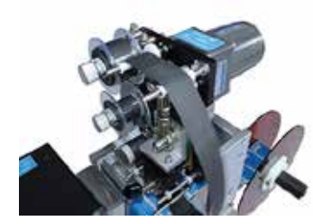
Dateur automatique qui assure l'impression sur l'étiquette grâce un encre à ruban
